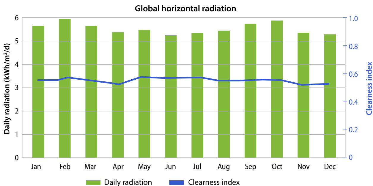
Fig. A4. Solar resource data for latitude 1.055, longitude 39.023
